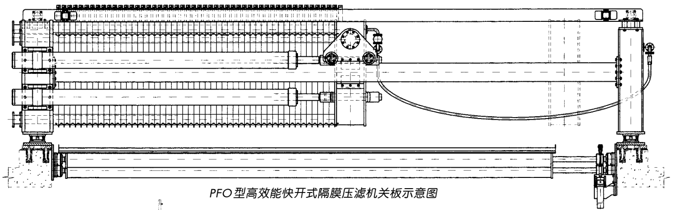
PFO 型高效能快开式隔膜压滤机开板示意图
