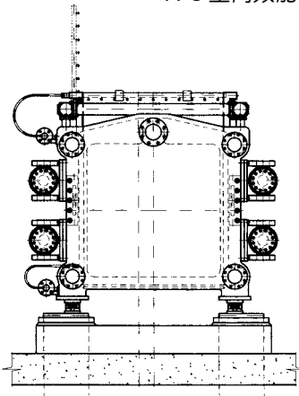
PFO 型高效能快开式隔膜压滤机关板示意图
